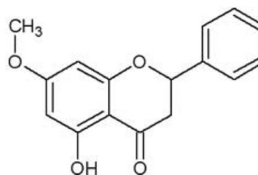
PINOSTROBIN
